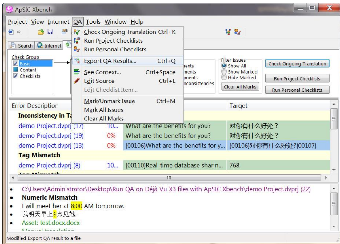
图 12 ApSIC Xbench 3.0 导出 QA 报告方法一
