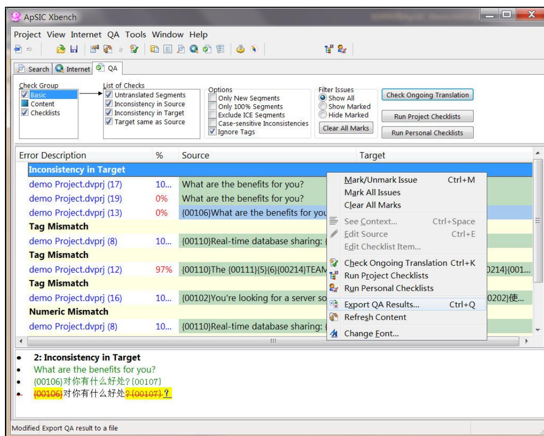
图 13 ApSIC Xbench 3.0 导出 QA 报告方法二
